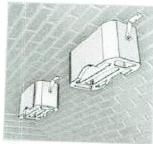
▲ Montaż sklepienia za pomocą regulowanego kątownika uchwytych
